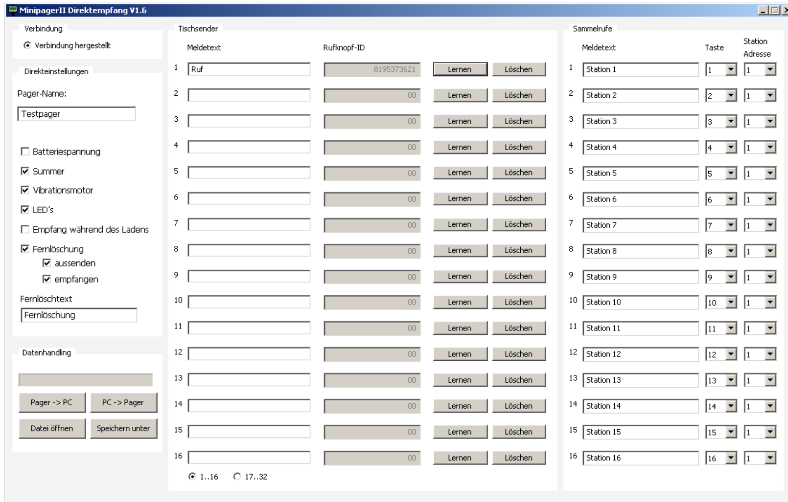
Abb.1: Bedienoberfläche "MP-T4_Direktempfang.exe"
